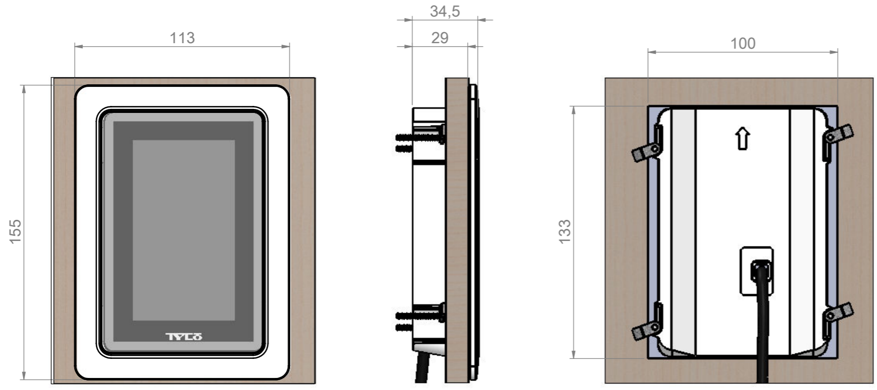
Cutout Dimensions
